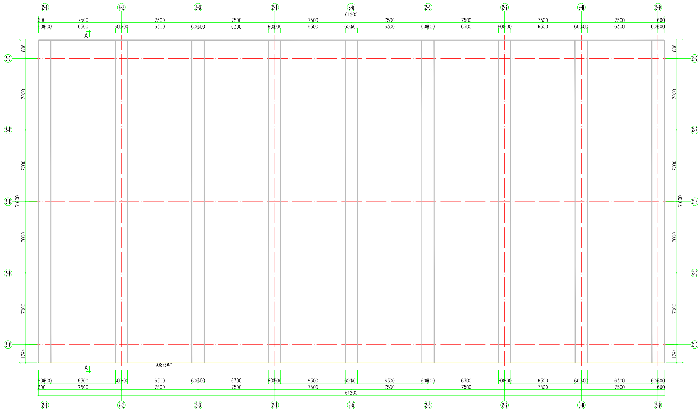
游泳馆屋面通杆结构平面布置图 1:100
